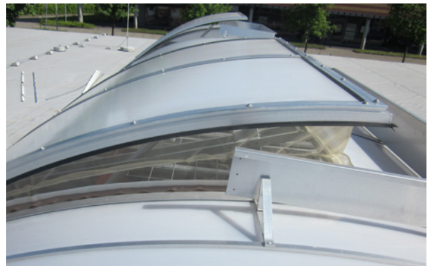
Lichtbandklappe in Lüftungsstellung mit Insektenschutzsystem
